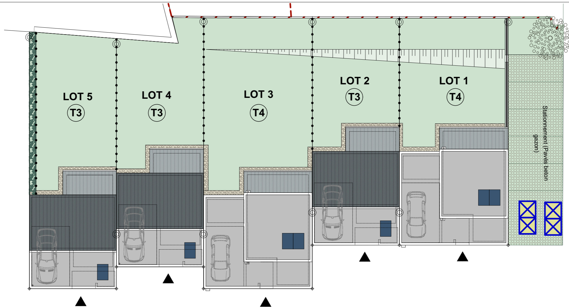
PLAN DE MASSE GÉNÉRAL ECH 1/200
