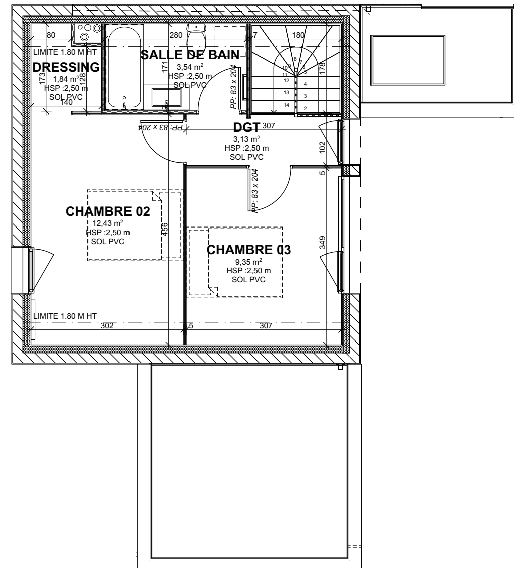
NIVEAU R+1 Ech: 1/75
