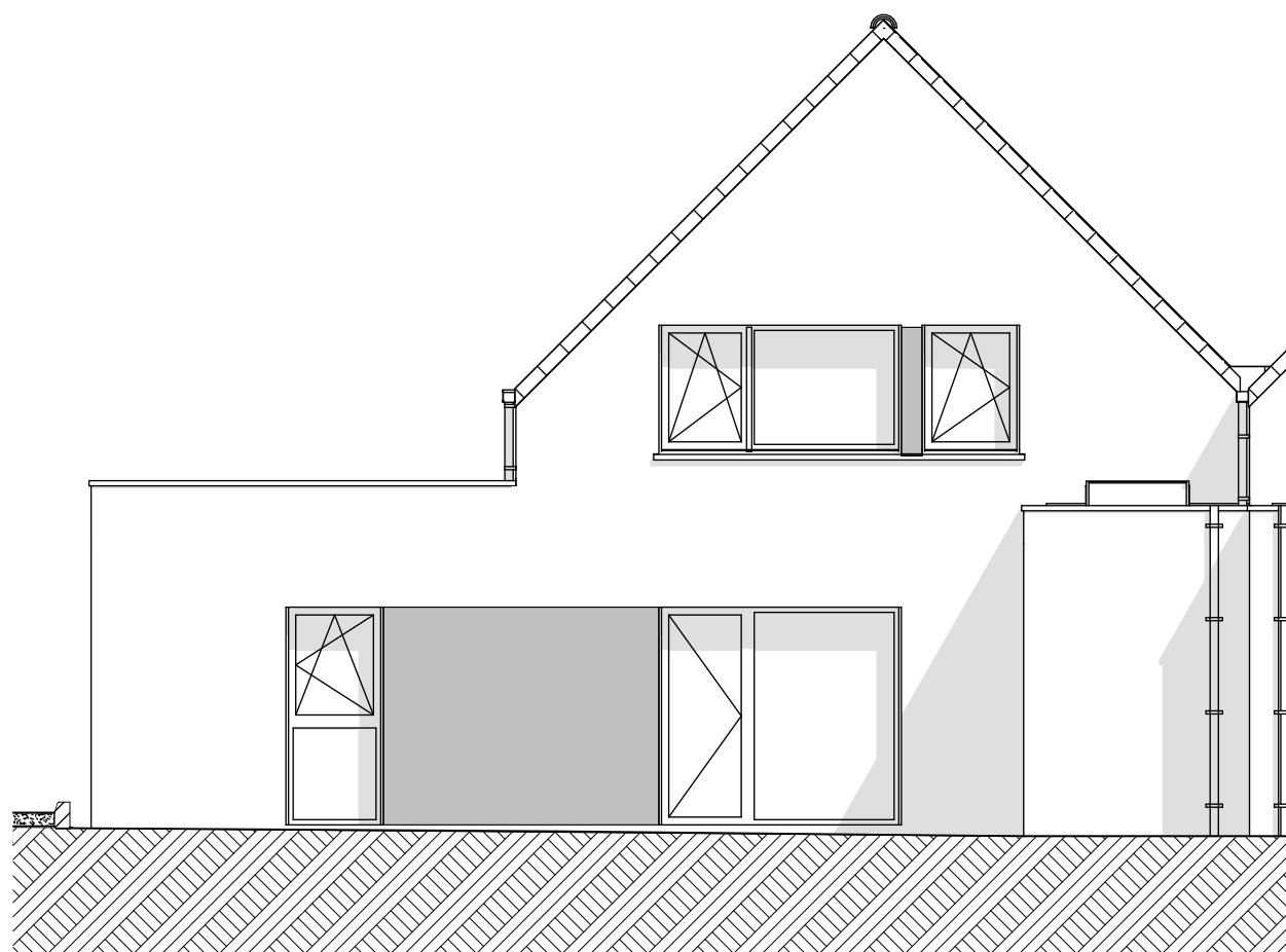
ELEVATION SUD EST Ech: 1/75
