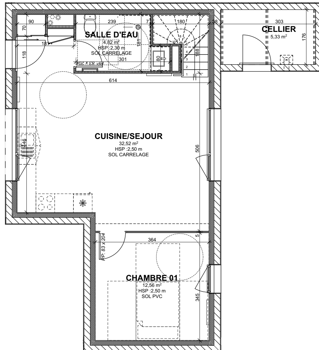
REZ-DE-CHAUSSEE Ech: 1/75
