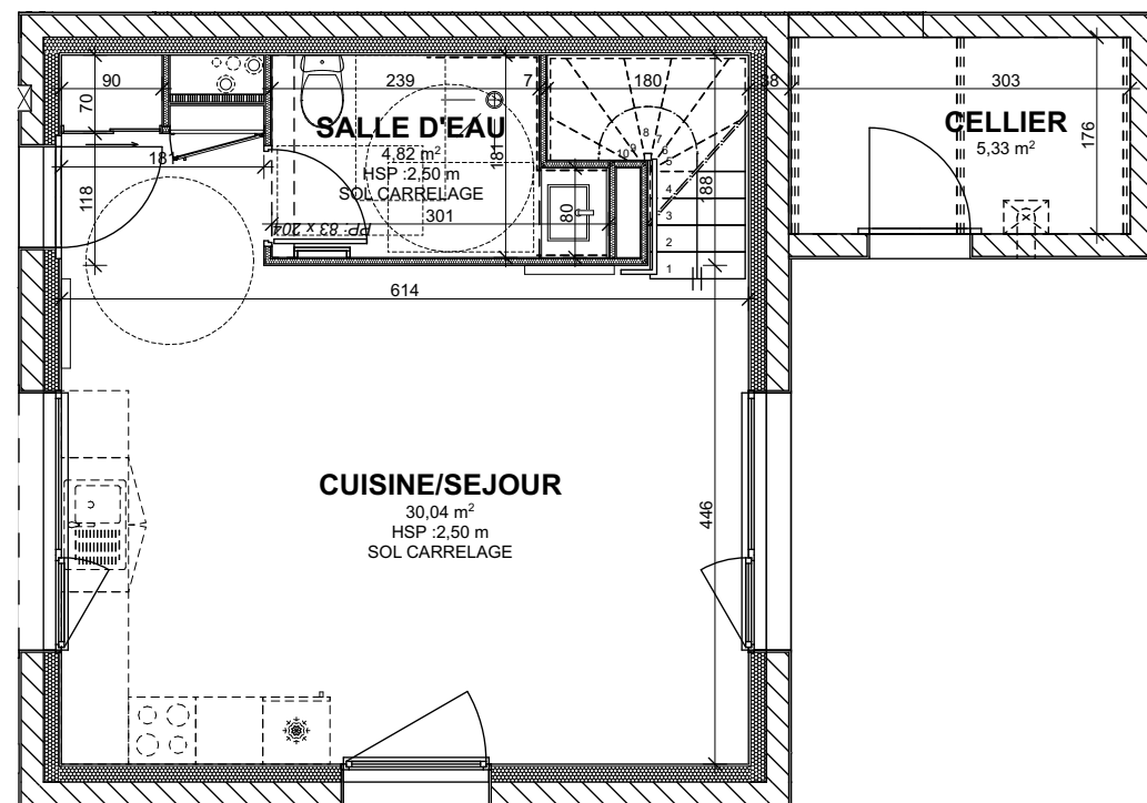
REZ-DE-CHAUSSEE Ech: 1/75
