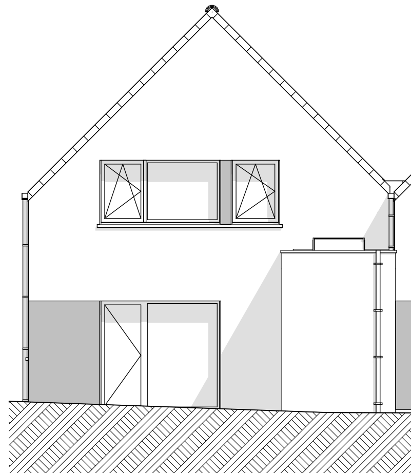
ELEVATION SUD EST Ech: 1/75
