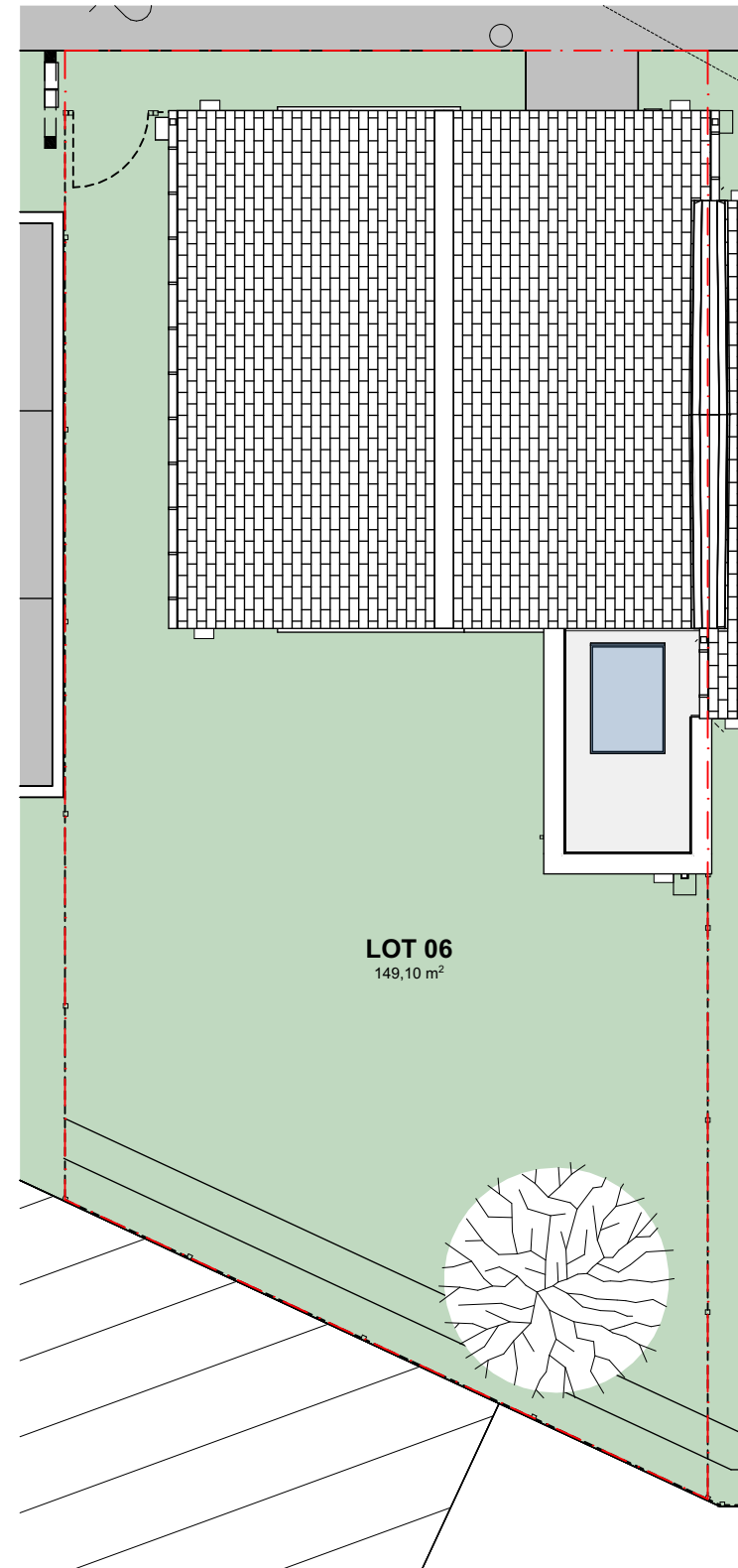
PLAN MASSE Ech: 1/100
