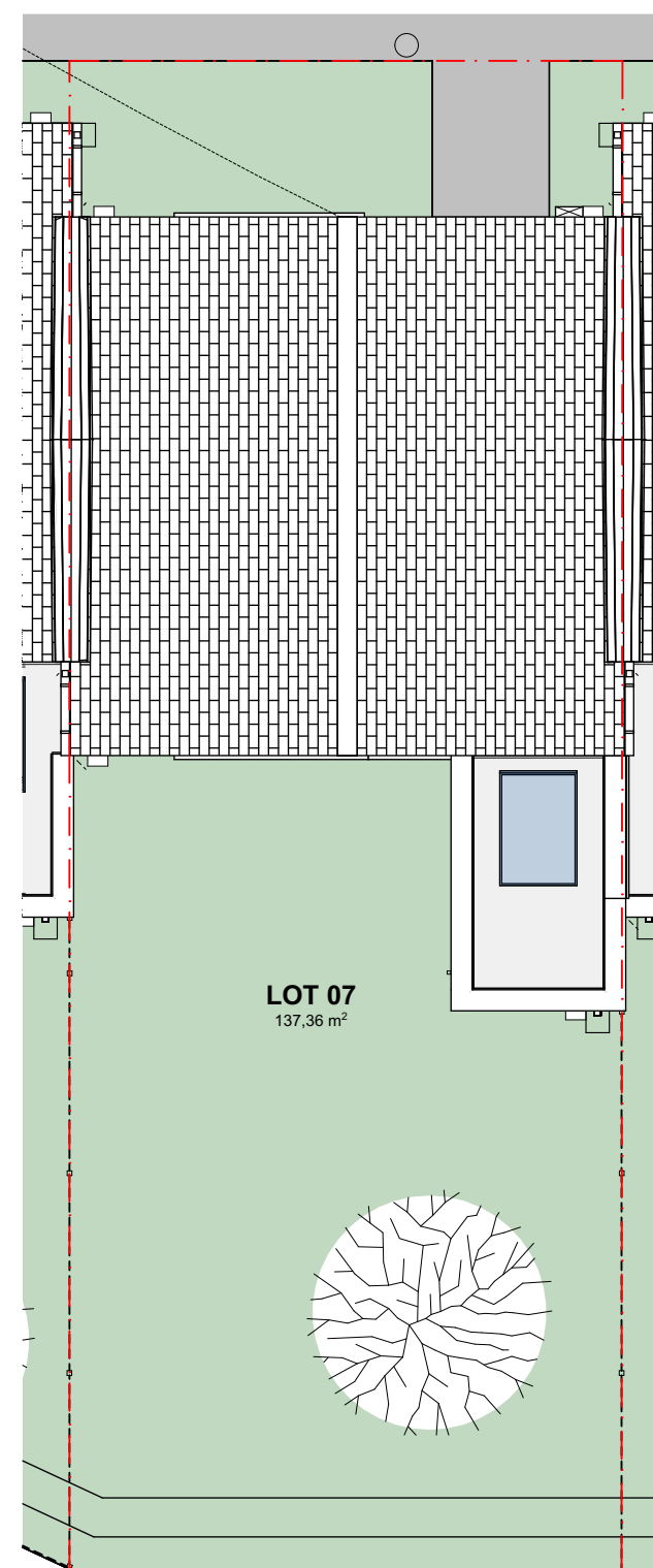
PLAN MASSE Ech: 1/100
