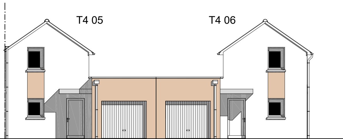
façade nord
