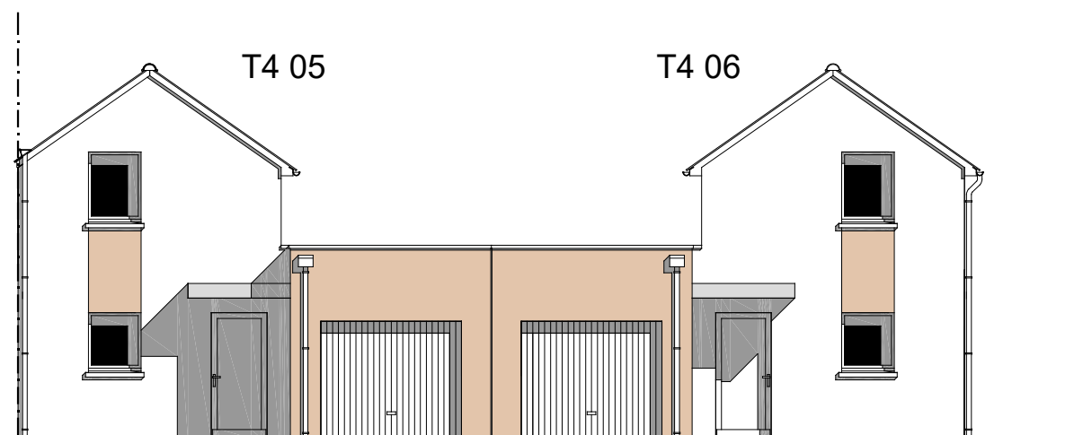
façade nord
