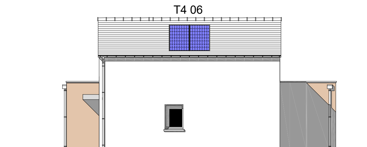
façade ouest
