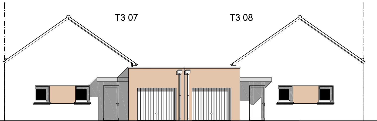
façade nord
