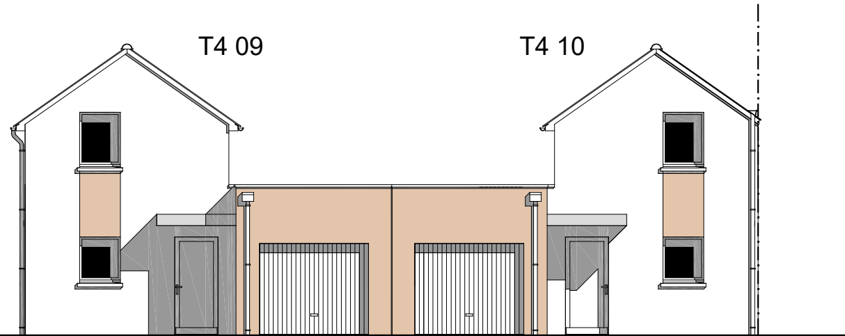
façade nord
