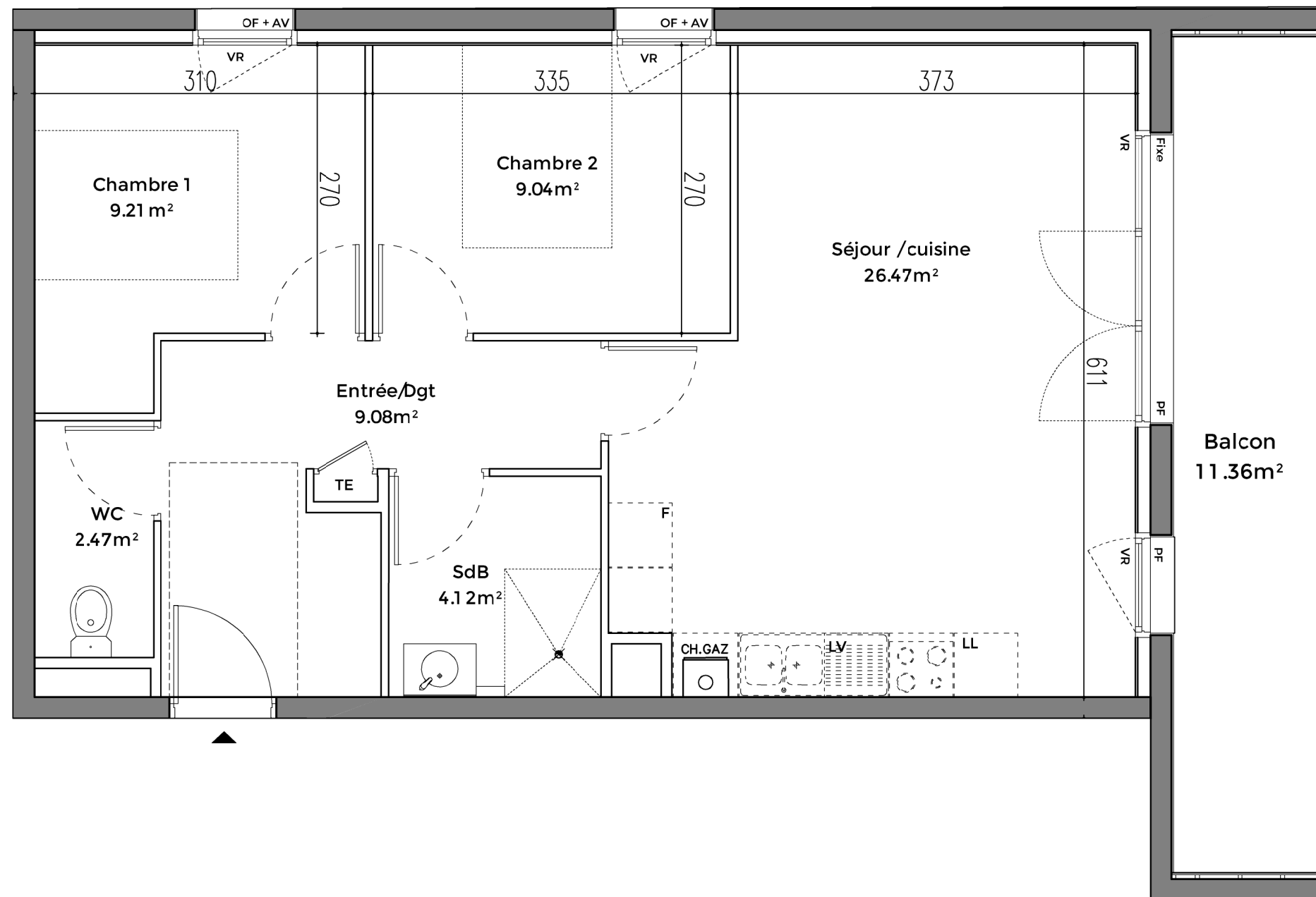
PLAN R+2
