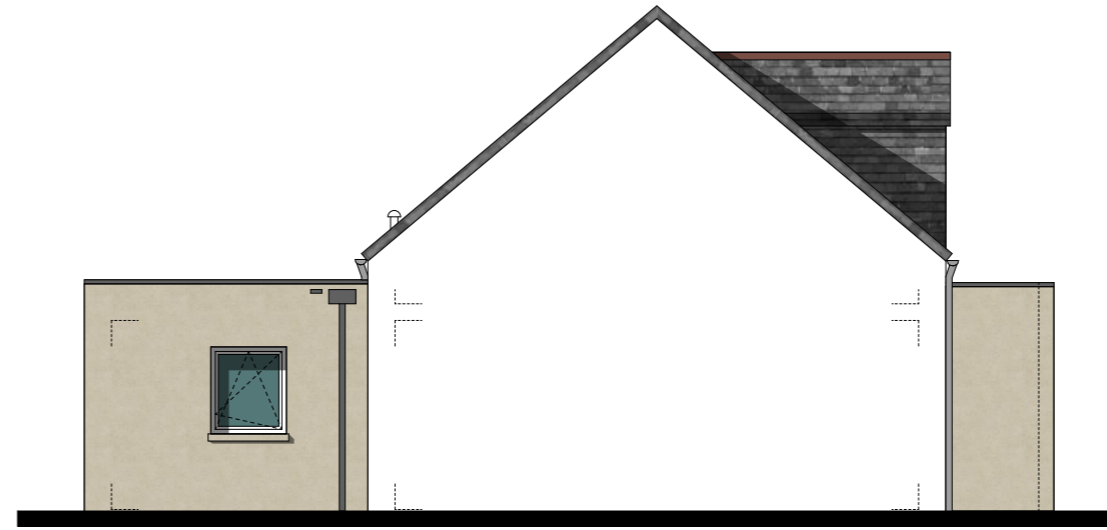
PIGNON OUEST
