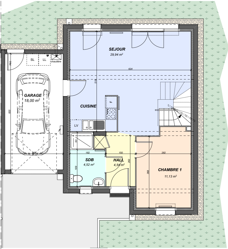
REZ-DE-CHAUSSÉE 50,14m²
