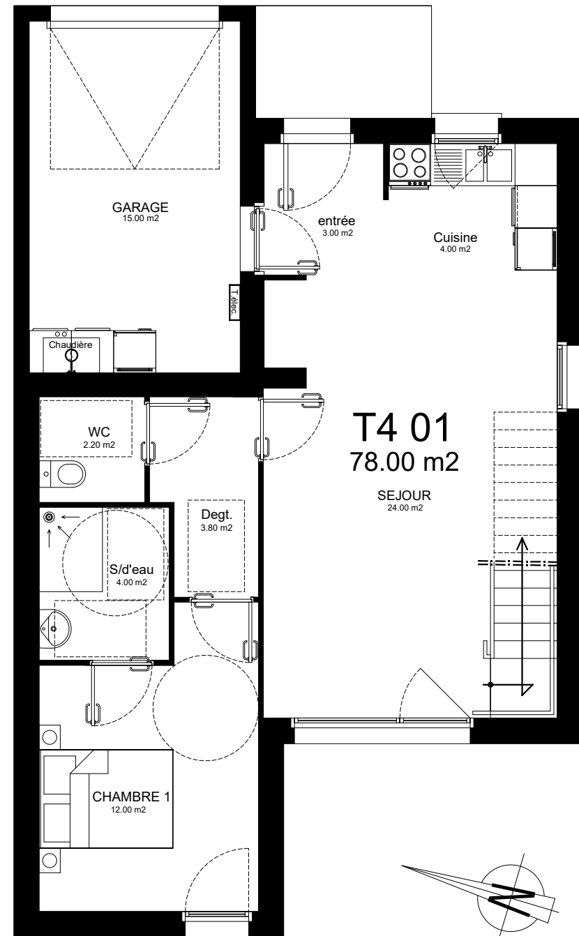
Rez de Chaussée
