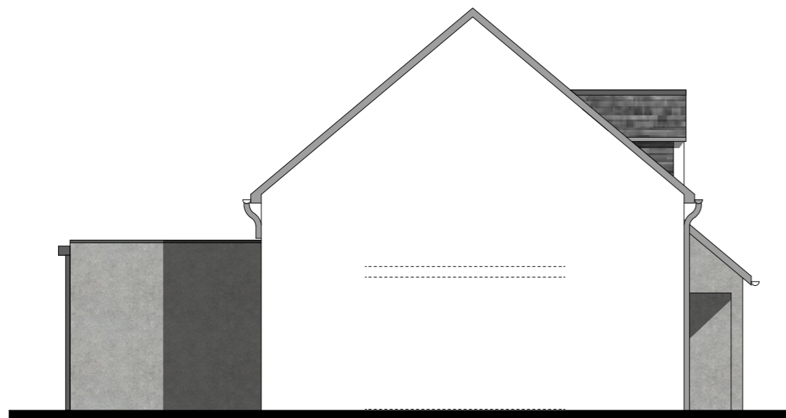
FACADE EST
