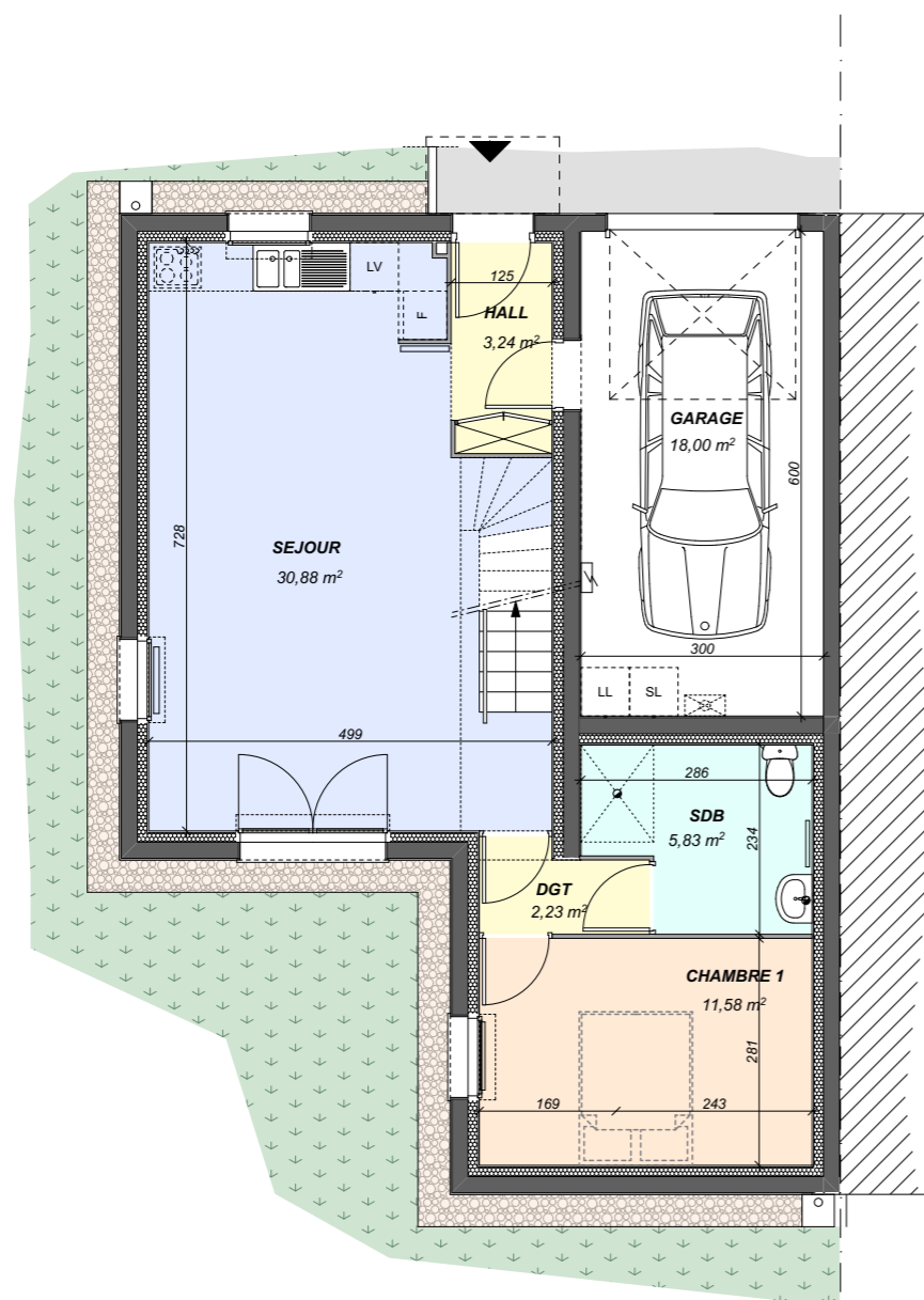
PLAN RDC 53,76m2
