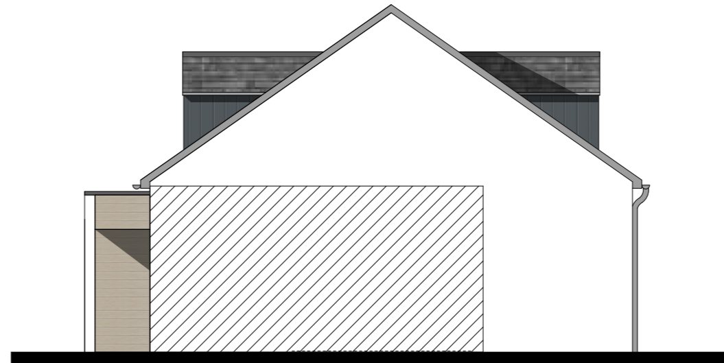
FACADE OUEST
