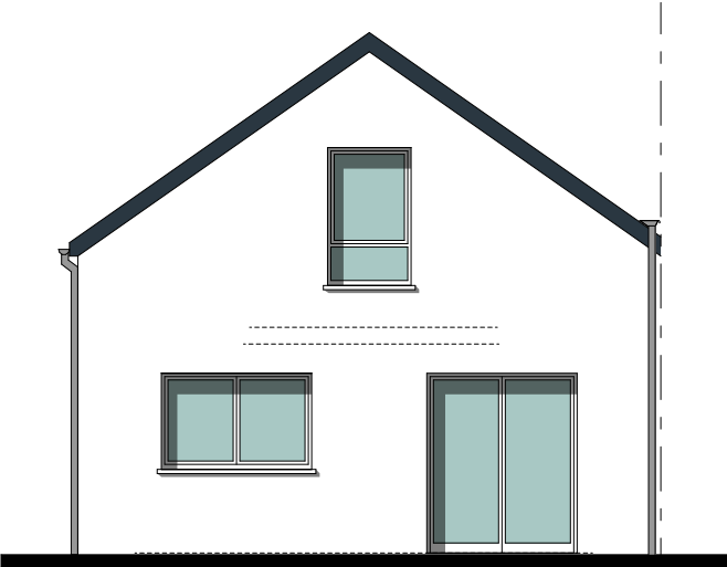
FACADE OUEST
