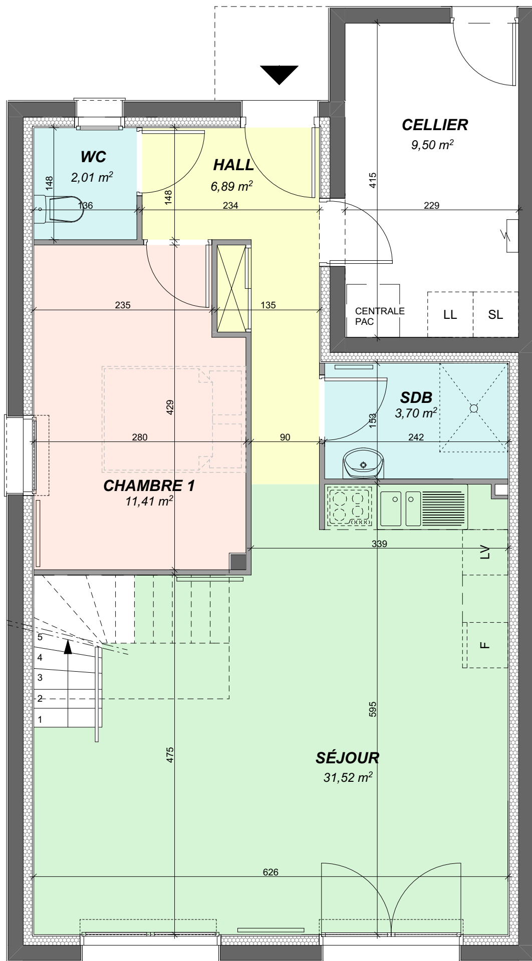
REZ-DE-CHAUSSÉE ECH 1/50
