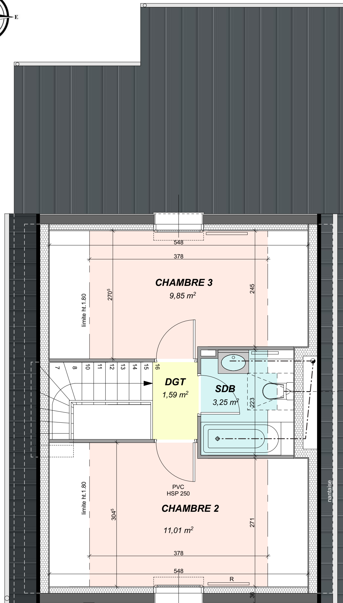
ÉTAGE ECH 1/50
