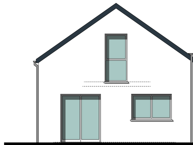
PIGNON SUD
