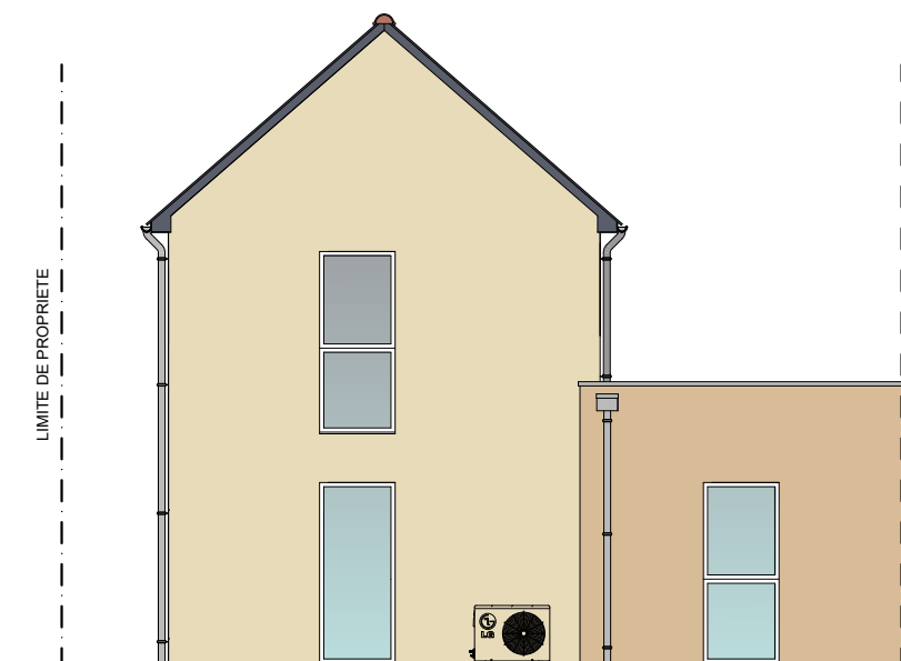
Façade Nord Est
