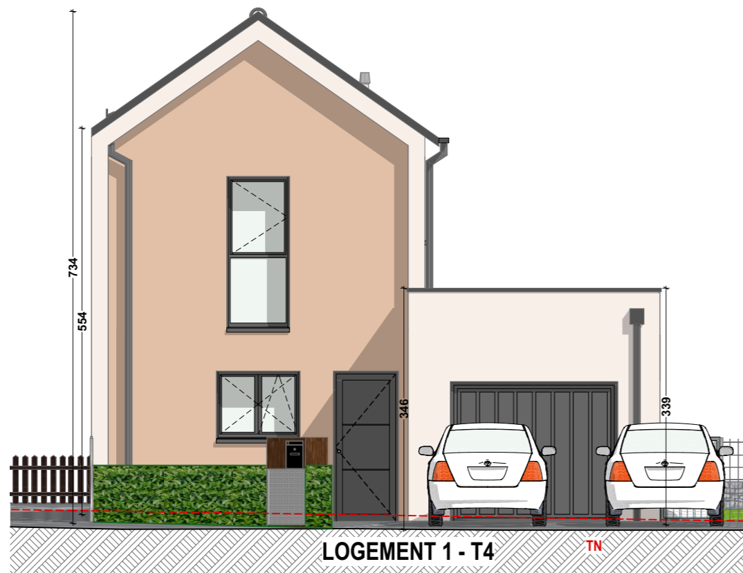
FACADE SUD ECH: 1/75 ème
